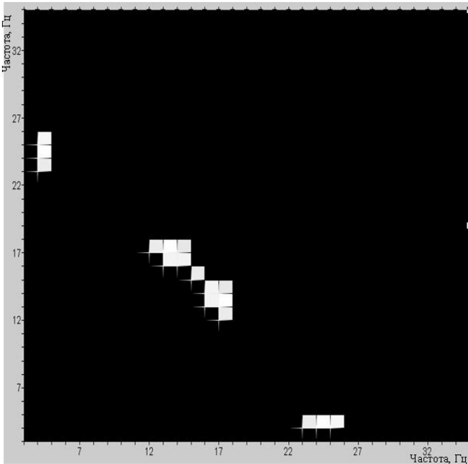
Рис. 5. Значения функции бикогерентности в отведении С4 у одного из испытуемых при репродукции сигналов длительностью 200 мс. На светлых участках функция бикогерентности \geq 0,8 , на темных – близка к нулю
