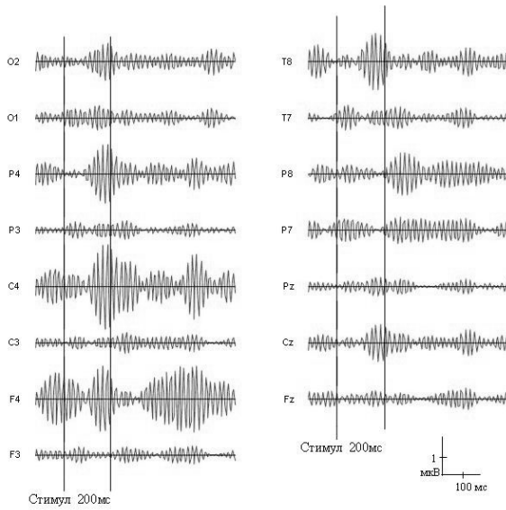
Рис. 2. Усредненные ССЭОМ при репродукции сигналов длительностью 200 мс в частотном диапазоне 30–70 Гц
