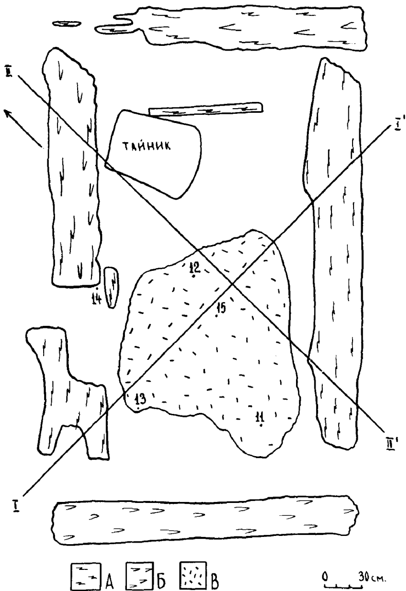
Рис. 3. Курган 53. План погребения.
