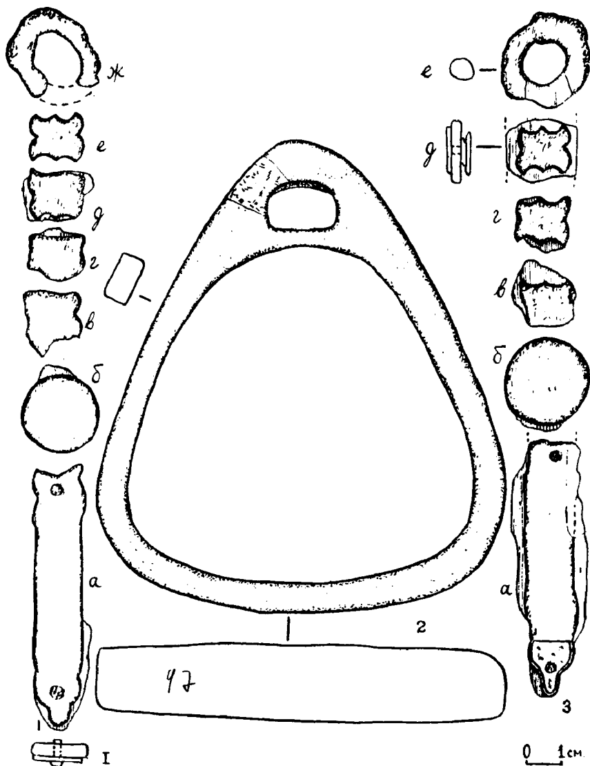
Рис. 8. Змеинкинский курганный мошльник. Курган 53. Тайник. Костяное стремя (2) и примыкающие к нему железные детали (1) путлищного ремня. Железные детали (3) второго путлищного ремня (без стремени). 2 - кость, остальное железо с остатками кожи.
