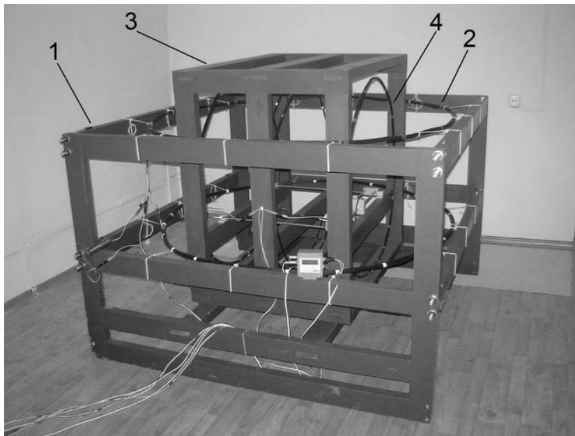
Рис. 1. Конструкция и внешний вид камеры: 1 – каркас соленоидов компенсации вертикальной составляющей ГМП; 2 – соленоиды компенсации горизонтальной составляющей ГМП; 3 – каркас соленоидов компенсации горизонтальной составляющей ГМП; 4 – соленоиды компенсации горизонтальной составляющей ГМП
