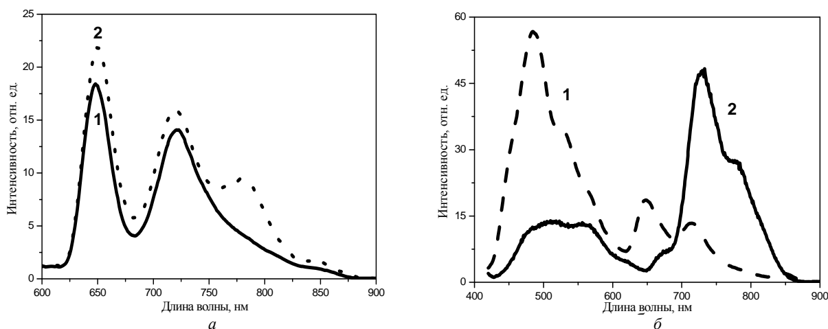
Рис. 2. Спектры долгоживущего излучения при 77К. а: \lambda_{\text{возб}} = 555 нм, 1 – H_2TPP-LuEDTA , 2 – H_2TPP-EDTA ; б: \lambda_{\text{возб}} = 400 нм, 1 – H_2TPP-DTPA , 2 – H_3TPP^+
