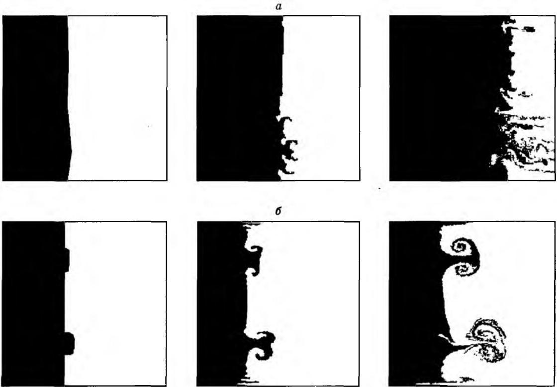
Рис. 15. Развитие неустойчивостей на границе двух сред: a — при слабом, b — при значительном возмущении профиля границы раздела.
