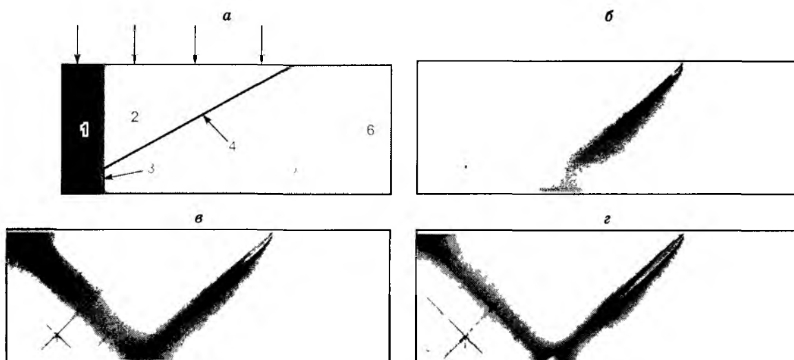
Рис. 12. Жесткие блоки 1 и 6 позволяют реализовать стесненную деформацию блоков 2 и 5 (блок 2 надвигается на блок 5, 4 — первичный разлом, схема а).
