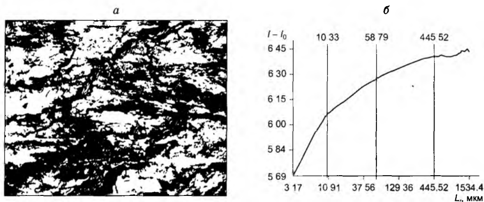
Рис. 1. Оптическое изображение излома угля (а) и характерные масштабы разрушения L_i \approx 10; 58; 445 мкм (б).
