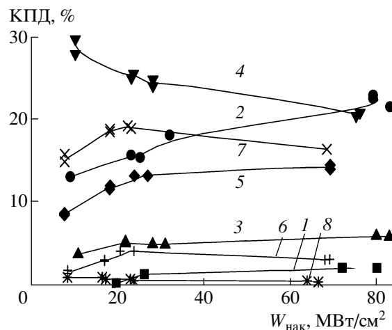
Рис. 6. Зависимости эффективности генерации твердотельных матриц с Ф512 (1–4) и P101T (5–8) от интенсивности возбуждения излучением 2-й гармоники Nd:YAG-лазера; 1 – ТЭОС-матрица, 5 – ТЭОС + ВТЭОС (7 : 3)-матрица; 2, 6 – композиты с ПММА; 3, 7 – композиты с ПММА + \text{Yb}(\text{NO}_3)_3 ; 4, 8 – композиты с ПС.
