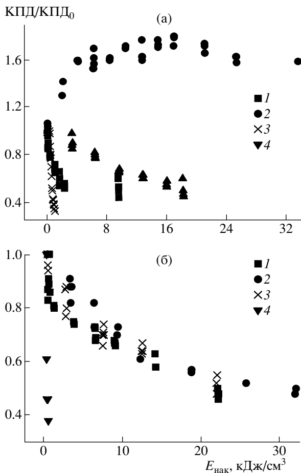
Рис. 7. Изменение эффективности генерации Ф512 (а) и P101T (б) в зависимости от суммарной поглощенной энергии возбуждения ( \lambda_{\text{возб}} = 532 нм) красителями в твердотельных матрицах: 1 (а) – ТЭОС; 1 (б) – ТЭОС + VTЭОС (7 : 3); 2 (а), 2 (б) – композиты с ПММА; 3 (а), 3 (б) – композиты с ПММА + \text{Yb}(\text{NO}_3)_3 ; 4 (а), 4 (б) – композиты с ПС.
