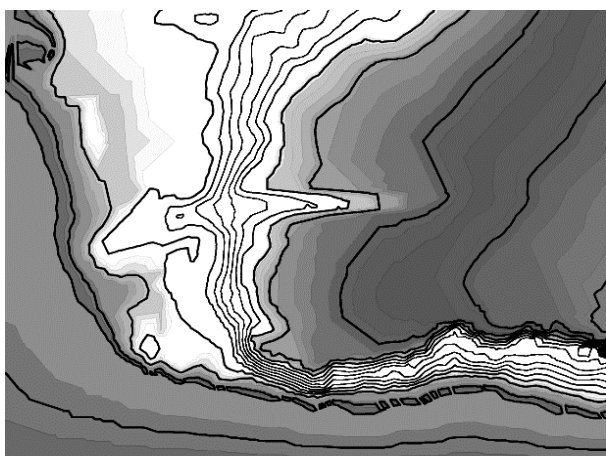
Рис. 2. Результат построения изоконтуров
