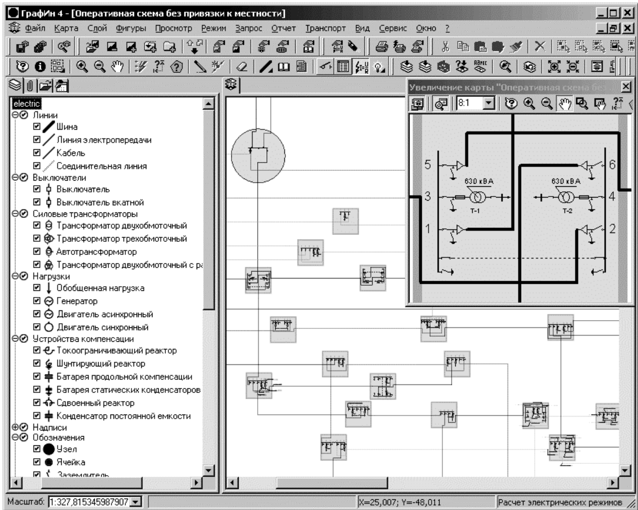
Рис. 2. Представление схемы электрической сети в ГИС Графин 4.0
