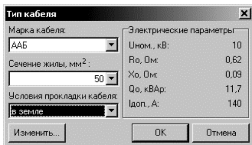
Рис. 4. Справочник кабелей
