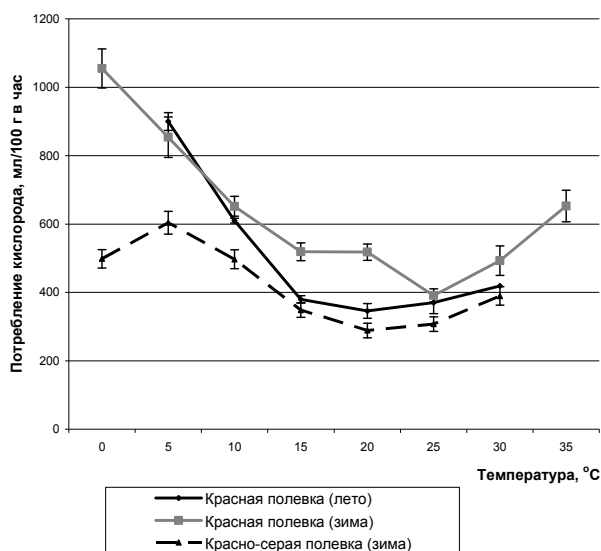
Рис. 1. Уровень обмена и химическая терморегуляция красной и красно-серой полевки
