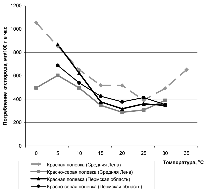
Рис. 2. Географические отличия химической терморегуляции красной и красно-серой полевков. Пермская область – по Н.В. Башениной [2]
