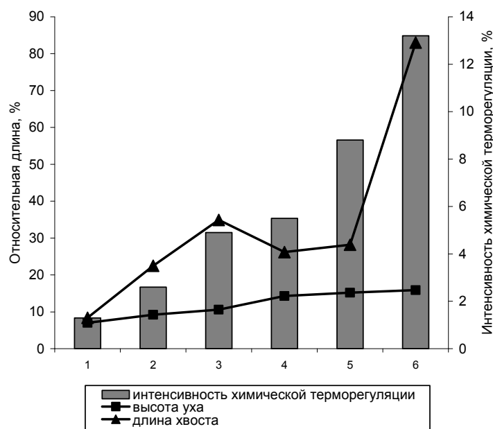
Рис. 4. Интенсивность химической терморегуляции и относительная длина выступающих частей тела у мелких млекопитающих: 1 – сибирский лемминг; 2 – северосибирская полевка; 3 – полевка-экономка; 4 – красно-серая полевка; 5 – красная полевка; 6 – домовая мышь
