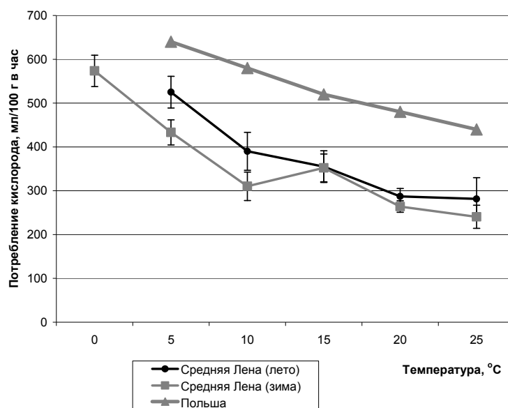
Рис. 3. Уровень обмена и химическая терморегуляция полевки-экономки. Польша – по Z. Gebczynska [15]
