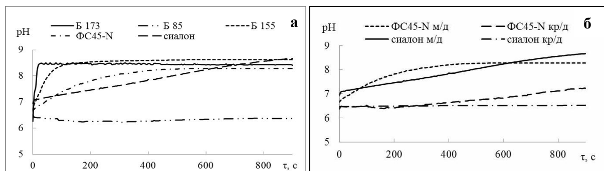
Рис. 1. Кинетические кривые изменения рН водных суспензий во времени: а – мелкодисперсных композитов, б – композитов в зависимости от дисперсности
