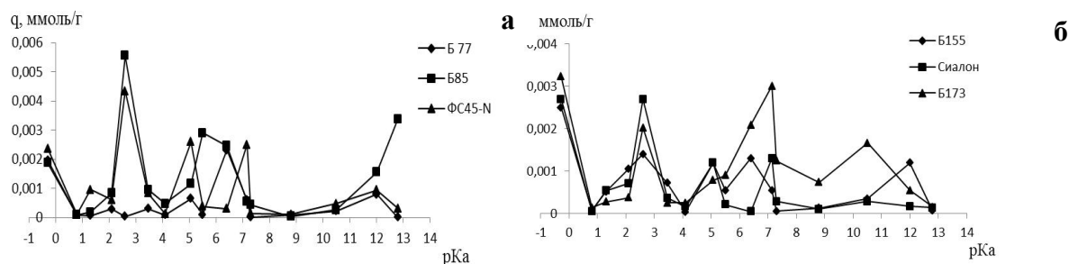
Рис. 2. Распределение центров адсорбции индикаторов на поверхности композитов: а – на основе нитрида кремния и смешанной основе, б – на основе нитрида бора и сиалона
