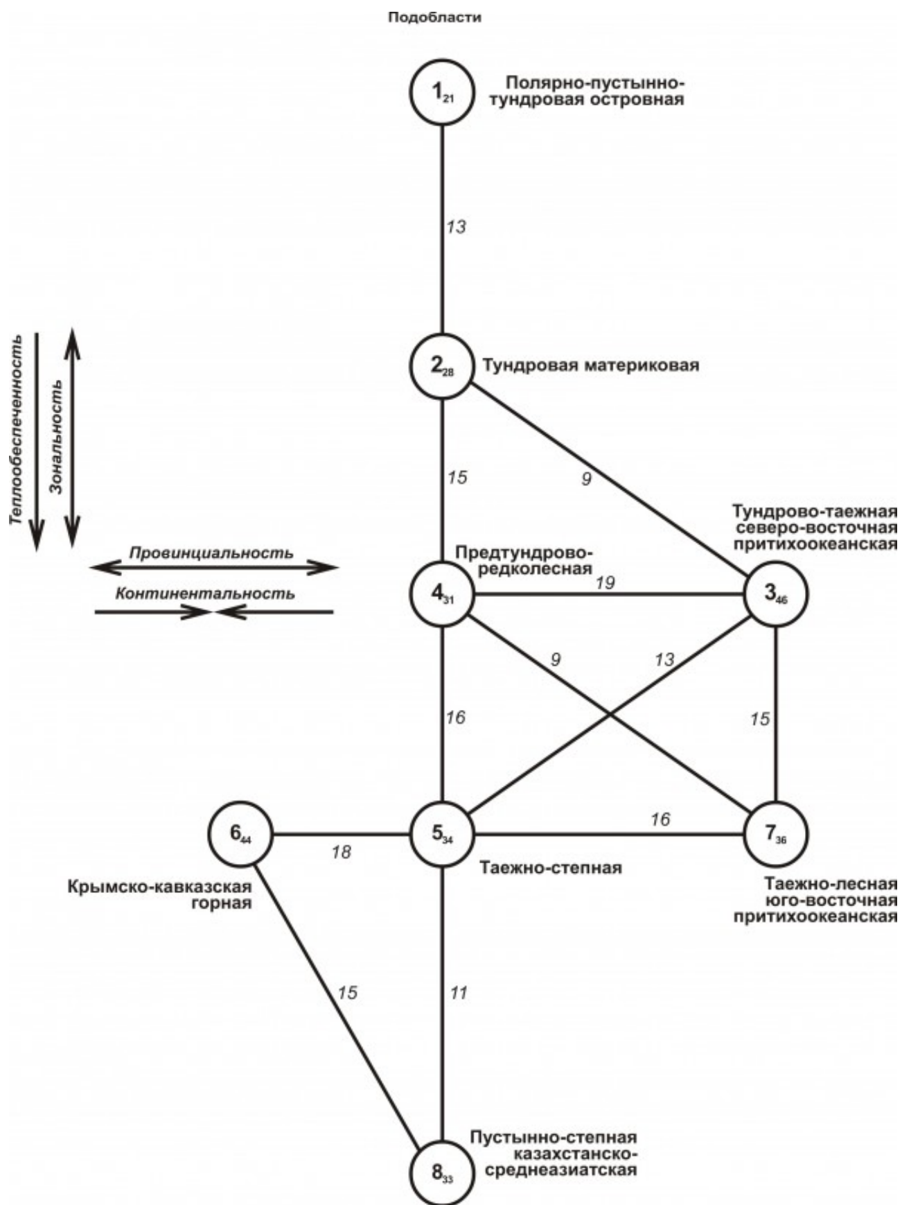
Рис. 2. Пространственно-типологическая структура флоры-фаунистической неоднородности Северной Евразии на уровне подобласти. Внутри значков приведены номера таксонов классификации (см. в тексте), в виде подстрочного индекса показана величина внутригруппового сходства. Между таксонами обозначена величина межгруппового сходства. Стрелки у перечня основных
