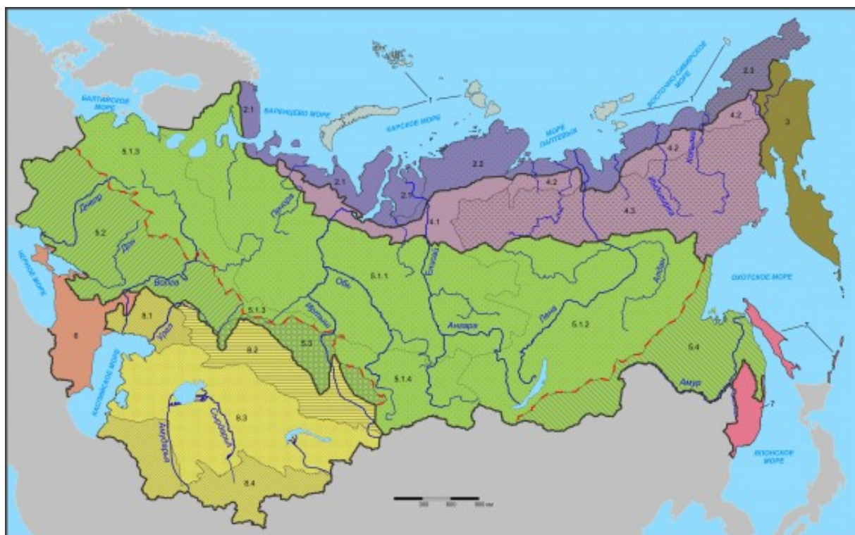
Рис. 1. Флоро-фаунистическое районирование Северной Евразии.
