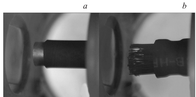
Рис. 1. Фотографии разрядного промежутка с анодом из стальной фольги (а) и вольфрамовых проволочек (b).
