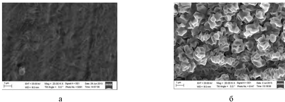
Рис.2. Морфология поверхности сплава ВТ-23 обработанного ионным пучком меди продолжительностью: 3 мин. (а) и 7,5 мин (б)
