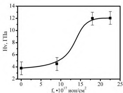
Рис.3. Зависимость микротвердости от флюенса облучения поверхностного слоя сплава ВТ-23 ионами меди
