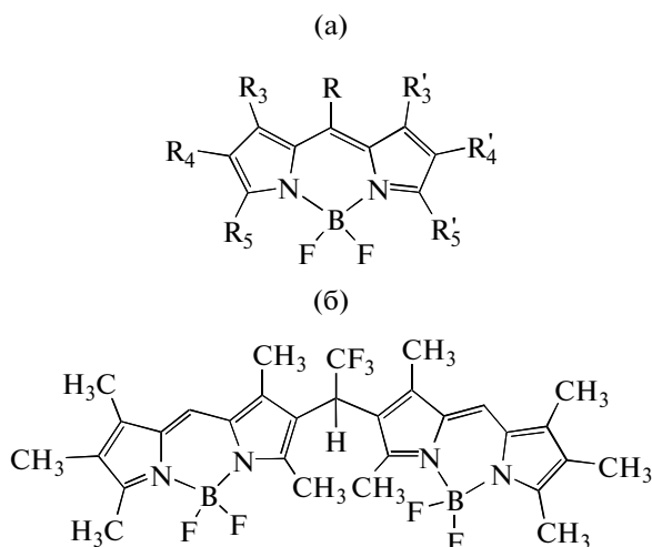
Рис. 1. Структурные формулы и обозначения исследованных BODIPY. а – BODIPY № 1: дифторборат 3,4,5-триметил-2,2'-дипирролилметена ( R_3 = R_4 = R_5 = R = H ; R_3 = R_4 = R_5 = CH_3 ); BODIPY № 2: дифторборат 3,3',5,5'-тетраметил-2,2'-дипирролилметена ( R = R_{4,4'} = H , R_{3,3'} = R_{5,5'} = CH_3 ); BODIPY № 3: дифторборат 3,3',5,5'-тетраметил-4,4'-диэтил-2,2'-дипирролилметена ( R = H , R_{3,3'} = R_{5,5'} = CH_3 , R_{4,4'} = C_2H_5 ); BODIPY № 4: дифторборат 3,3',5,5'-тетраметил-4,4'-диэтил- ms -фенил-2,2'-дипирролилметена ( R_{3,3'} = R_{5,5'} = CH_3 , R_{4,4'} = C_2H_5 , R = C_6H_5 ); BODIPY № 5: дифторборат 3,3',5,5'-тетраметил-4,4'-дибензил-2,2'-дипирролилметена ( R_{3,3'} = R_{5,5'} = CH_3 , R_{4,4'} = CH_2-C_6H_5 , R = H ); BODIPY № 6: дифторборат 3,3',5,5'-тетрафенил-2,2'-дипирролилметена ( R_{3,3'} = R_{5,5'} = C_6H_5 , R_{4,4'} = R = H ); BODIPY № 7: дифторборат мезо -пропаргиламино-2,2'-дипирролилметена ( R_{3,3'} = R_{4,4'} = R_{5,5'} = H , R = NH-CH_2-C\equiv CH ); б – BODIPY №8: бис -дифторборат бис(1,2,3,7,9-пентаметил-8-ил-дипирролилметен) ms -трифторметана.
