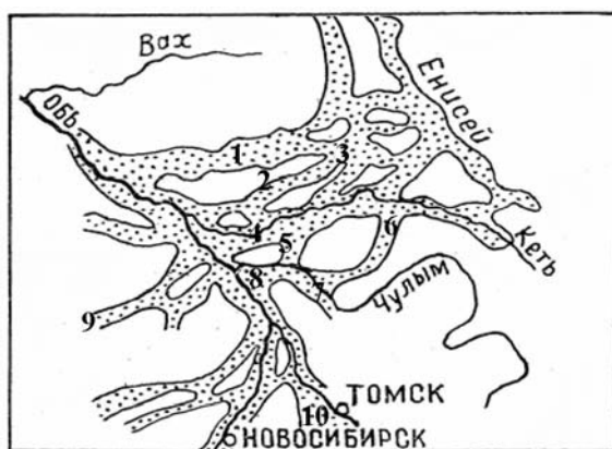
Рис. 4. Ложбины древнего стока [11, 12]: 1 – Тымская; 2 – Пайдугинская; 3 – Орловская; 4 – Кетская; 5 – Нибегинская; 6 – Улулюльская; 7 – Малоюксинская и Большеюксинская; 8 – Лайская; 9 – Чузикская; 10 – Чернореченская
