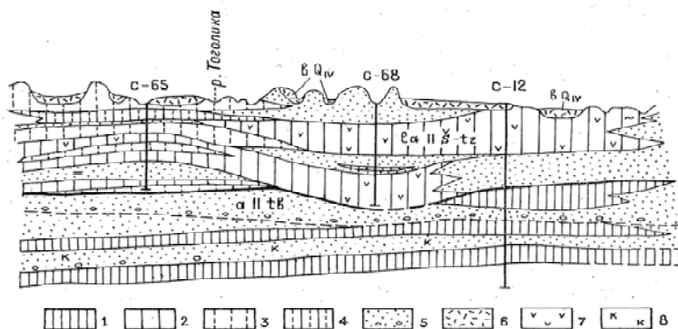
Рис. 2. Геологический разрез Кеть-Тымского междуречья [12]: 1 – глины; 2 – суглинки; 3 – супеси; 4 – переслаивание суглинков, супесей; 5 – пески разнородные с гравием и галькой; 6 – торф; 7 – растительный детрит; 8 – каолинизация
