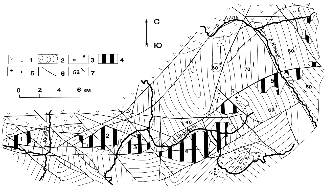
Рис. 1. Схема размещения расслоенных мафит-ультрамафитовых массивов нижнедербинского комплекса (составлена А.Г. Еханиным и др., 1991): 1, 2 – вмещающие породы: 1 – среднепалеозойские вулканогенно-осадочные (быскарская серия) Северо-Минусинской котловины, 2 – нижнепротерозойские карбонатно-сланцевые (дербинская свита) Дербинского антиклинория; 3 – среднепалеозойские гранитоиды; 4 – мафит-ультрамафитовые массивы (1 – Аштатский, 2 – Азертаский, 3 – Нижнедербинский, 4 – Бурлакский, 5 – Конжульский); 5 – позднепротерозойские гранитоиды; 6 – разрывные нарушения; 7 – элементы залегания слоистости
