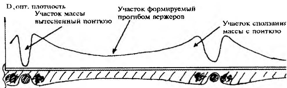
Рис. 2. Усредненная кривая распределения оптической плотности бумаги на интервале между двумя понтюзо
