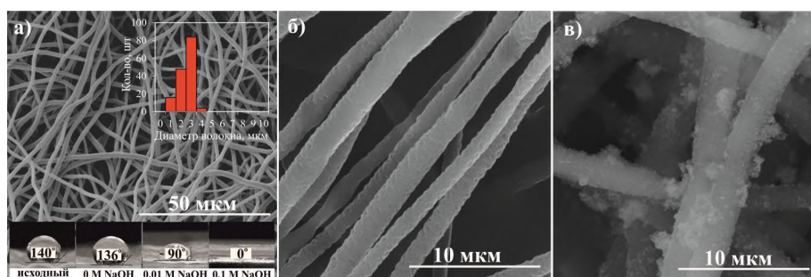
Рис. 1. Типичные СЭМ изображения матрицы ПМК и контактный угол смачивания при различных концентрациях NaOH (а), волокна ПМК без обработки НЧ ZnO (б) и с обработкой (в)
